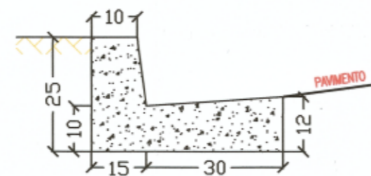
MEIO FIO COM SARJETA ESC: S/ESCALA Medidas em centímetros
