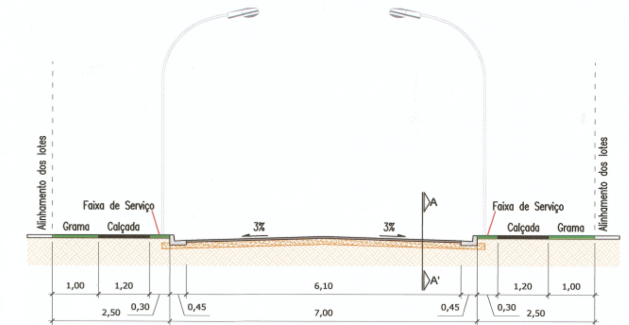
DETALHE SEÇÃO TRANSVERSAL ESC: S/ESCALA
