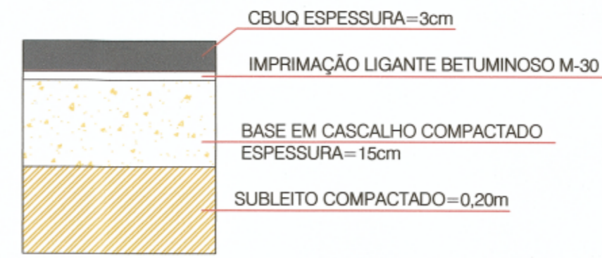
DETALHE SEÇÃO DO PAVIMENTO ESC: S/ESCALA
