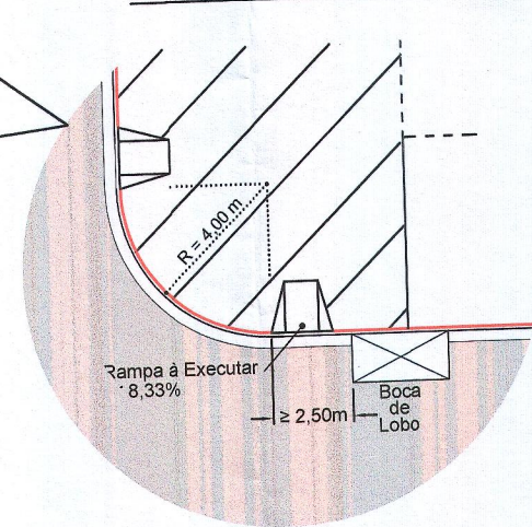
DETALHE RAIOS DA CURVA
