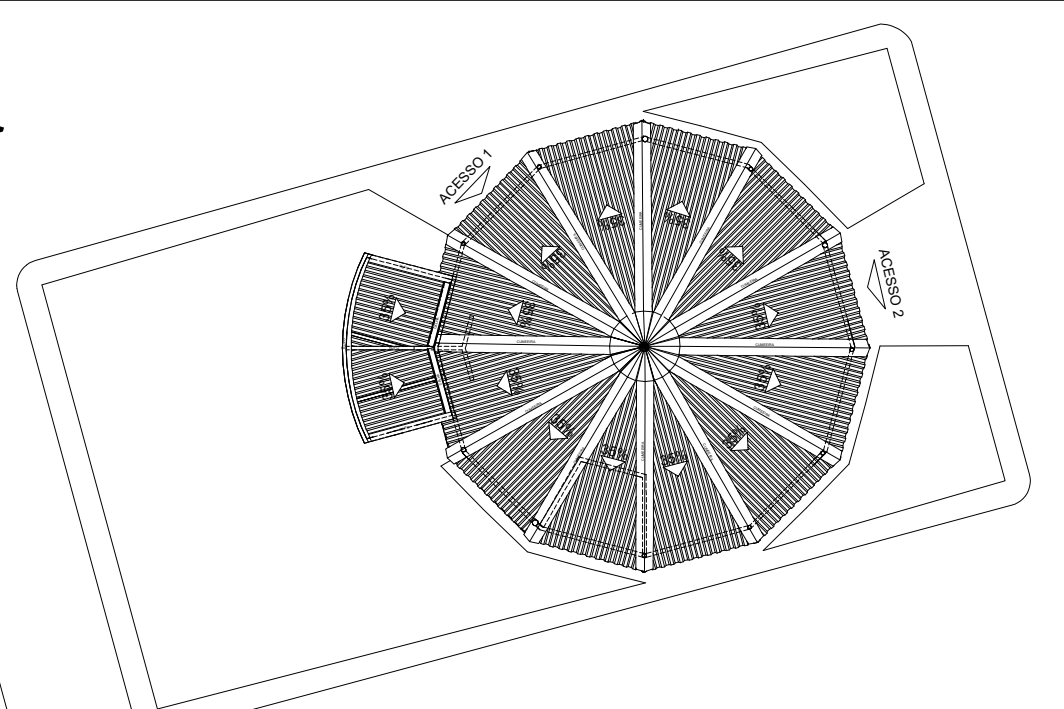
IMPLANTAÇÃO ESC.: 1/300
