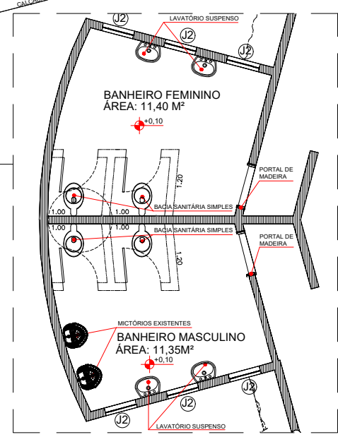
PLANTA ATUAL - BANHEIROS ESC.: 1/100
